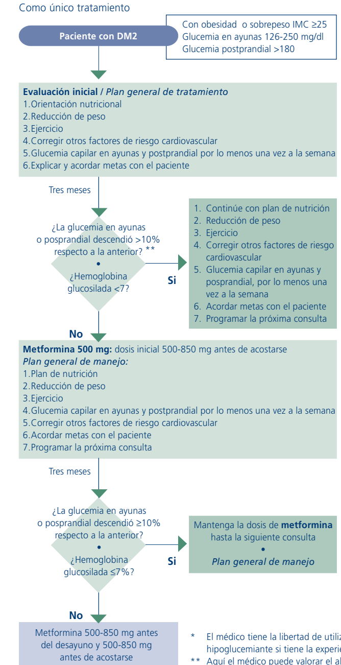
FIGURA 3. METFORMINA
